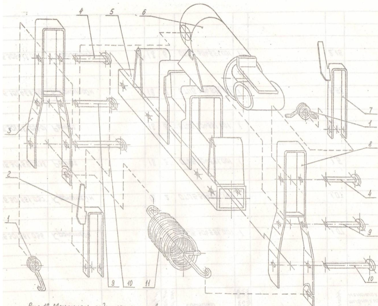
Рисунок 26 Механизм подъема маркеров ОТИБ.304551.001 (или маркер ОТИБ.305449.007 с гидроцилиндром Ц50-3405215 и гидроуправляемым распределителем)
