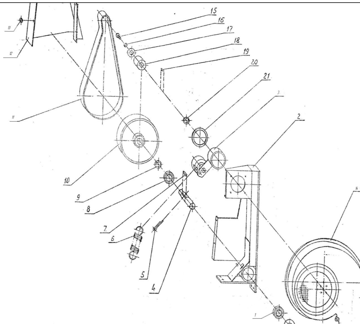
Рисунок 10 Привод вентилятора ОТИБ.303352.001
