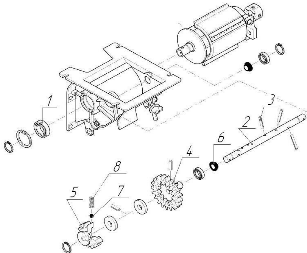
Рисунок 2 Узлы аппарата высевающего
