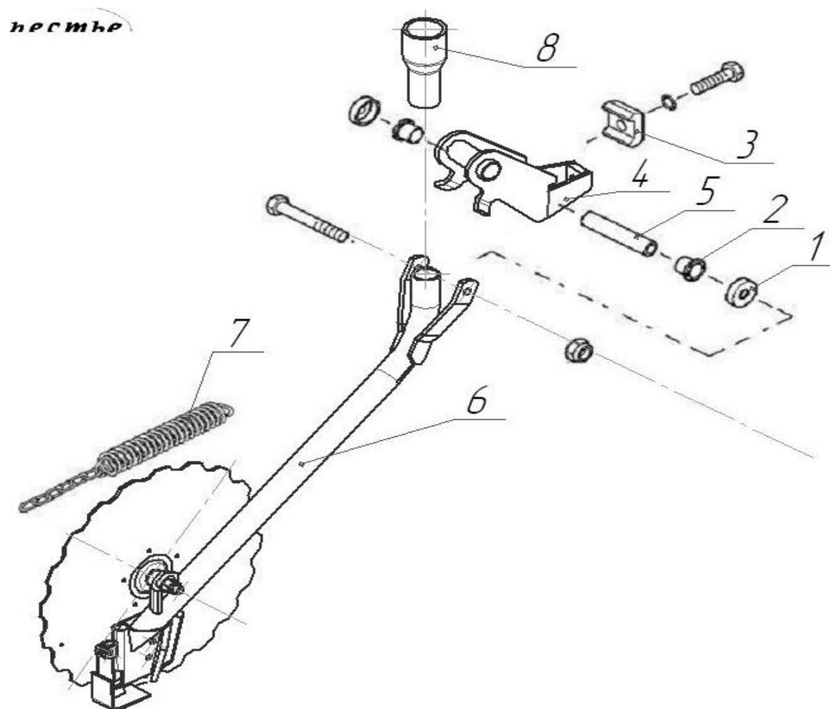
Рисунок 19 Крепление сошника заднего
