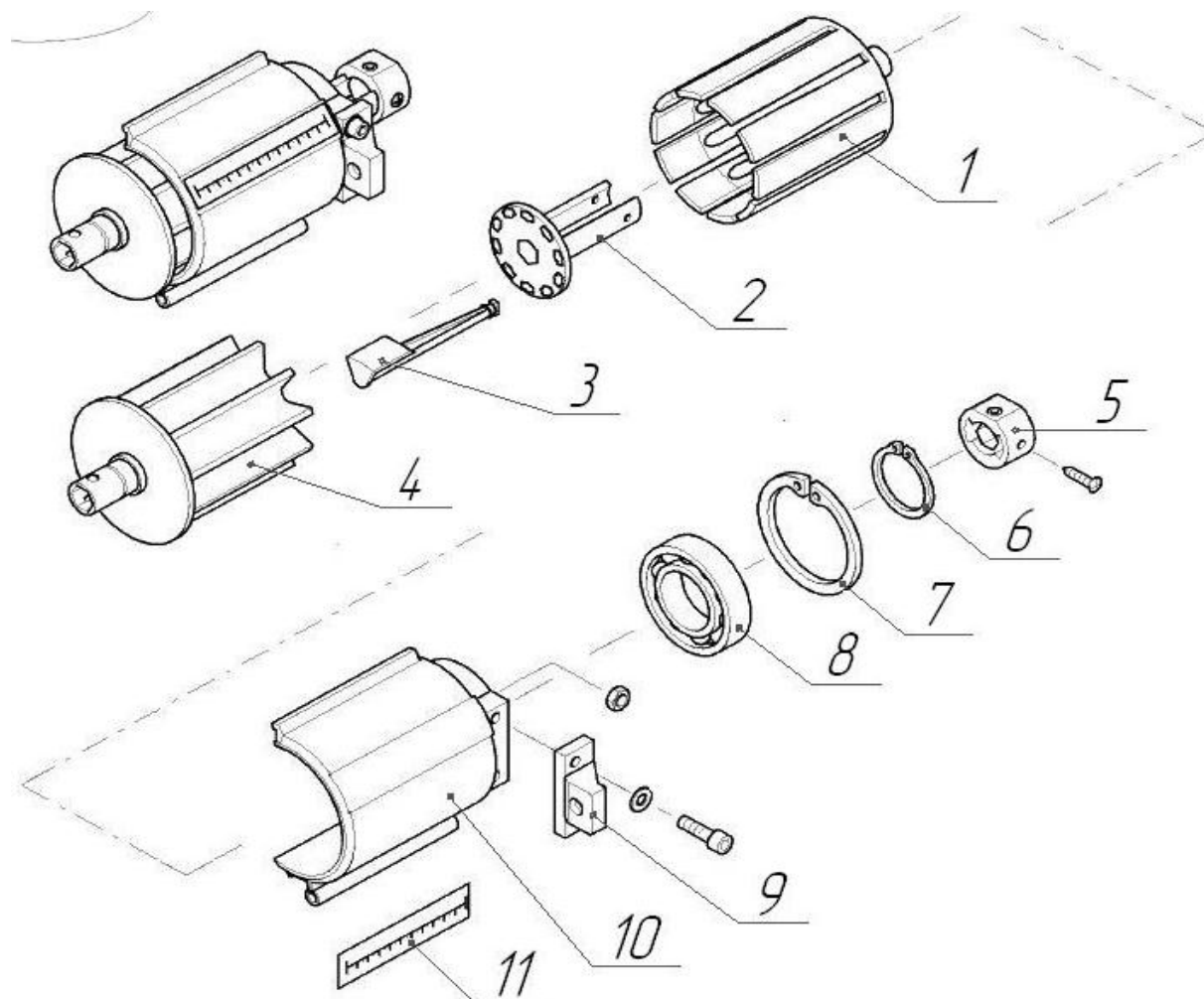
Рисунок 4 Узлы аппарата высевающего
