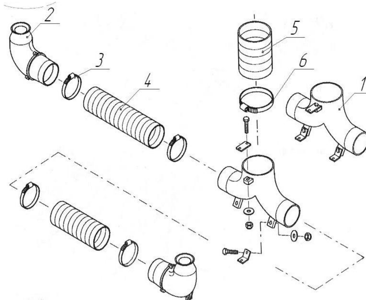
Рисунок 9 Узлы на соединение воздуховода
