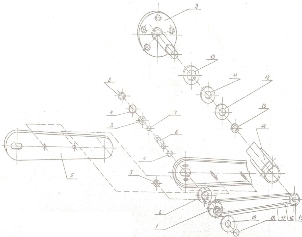
Рисунок 11 Опора ОТИБ.301235.003
