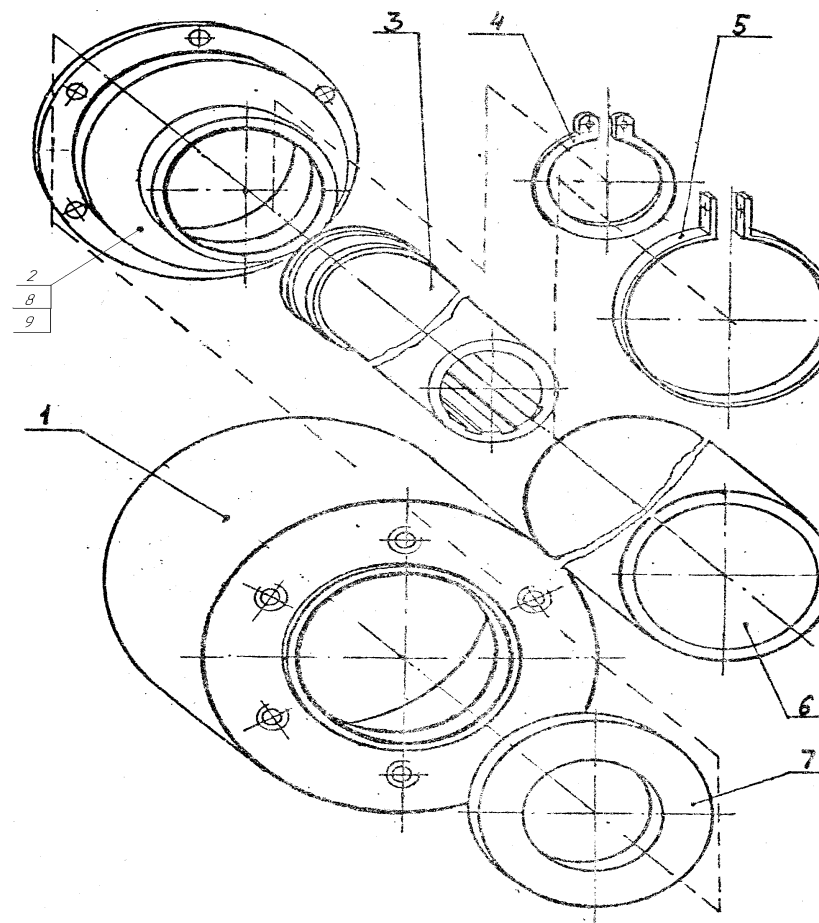
Рисунок 22 Вал карданный ОТИБ.303714.007-02
